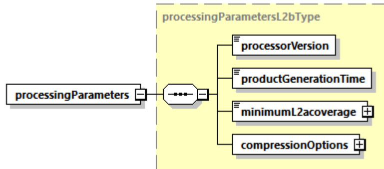
Fig.22 processing parameters L2b DSR
